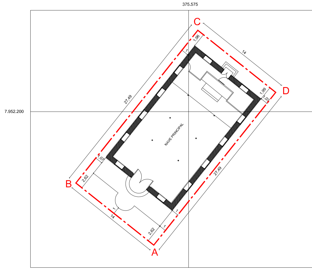
PLANO DE LÍMITES ESCALA GRÁFICA 0 5 10 15 m
