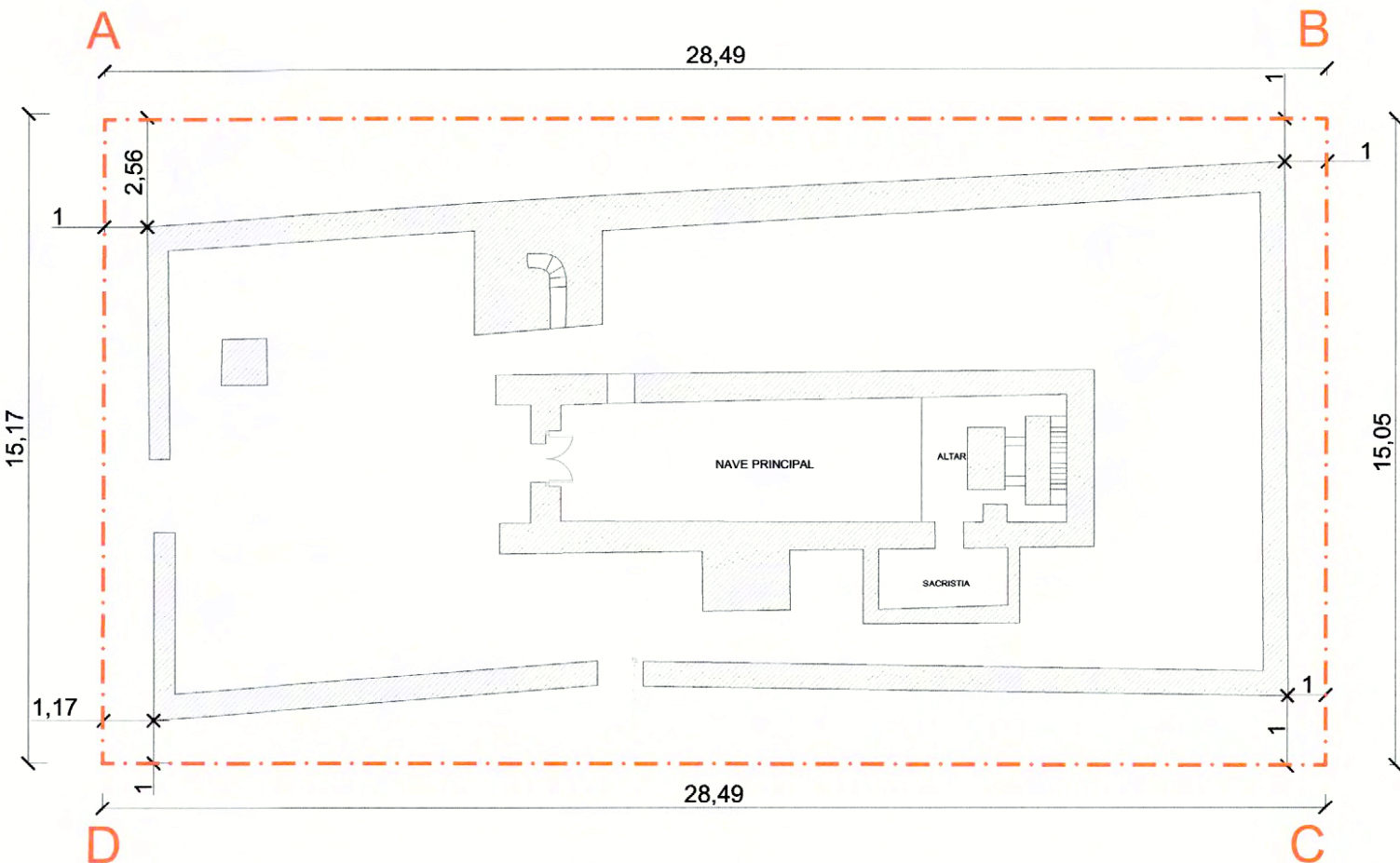
PLANO DE LÍMITES escala 1:200
