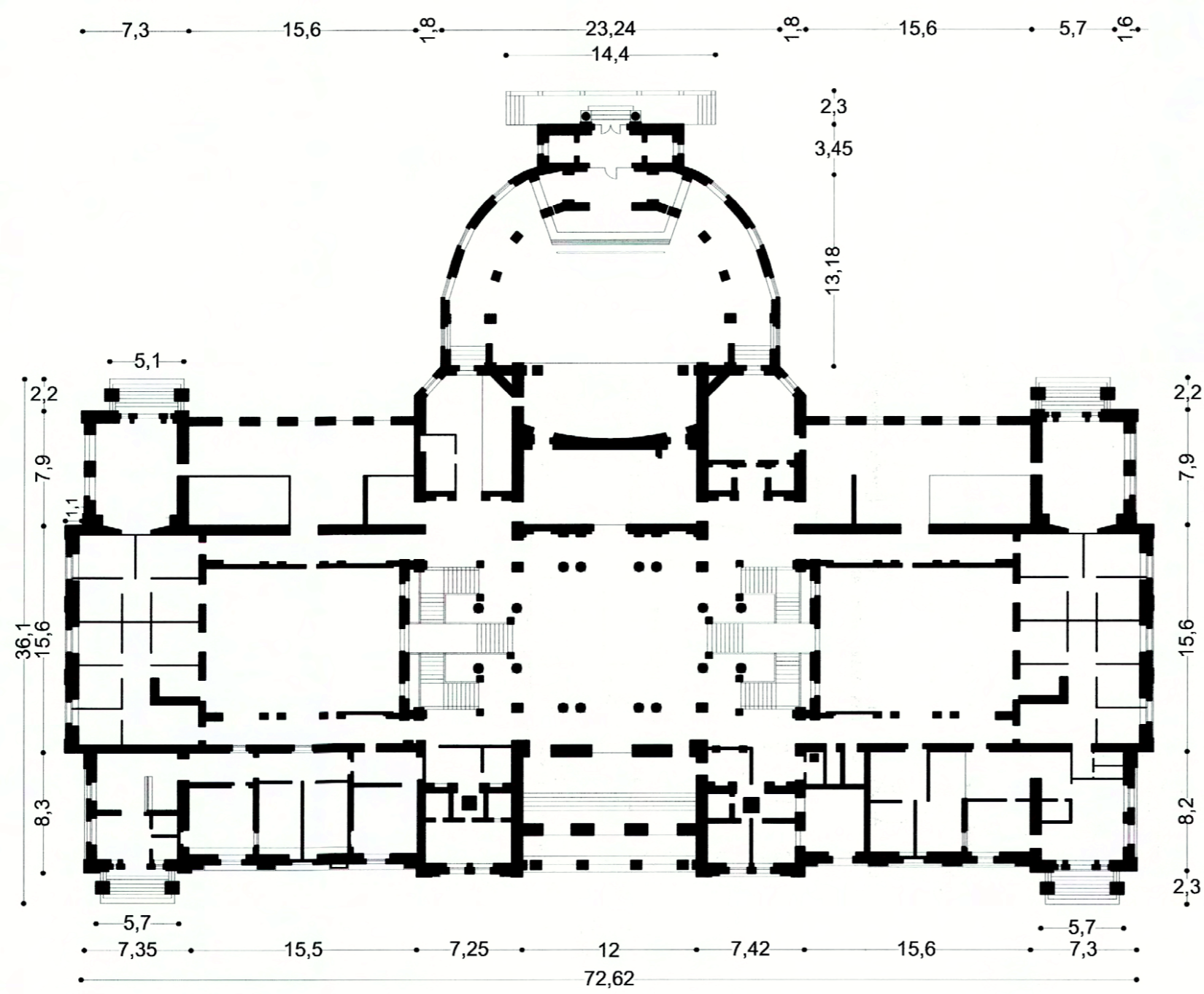
PLANTA GENERAL 0 5 10 15 20 m
